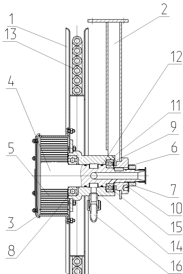
1- барабан; 2- кронштейн; 3- крышка; 4- вал; 5- пружина; 6- шайба стопорная; 7- гайка; 8,9- подшипник; 10- шпонка; 11- кольцо защитное; 12- кольцо; 13- РВД; 14- ступица барабана; 15- ось; 16- труба.
