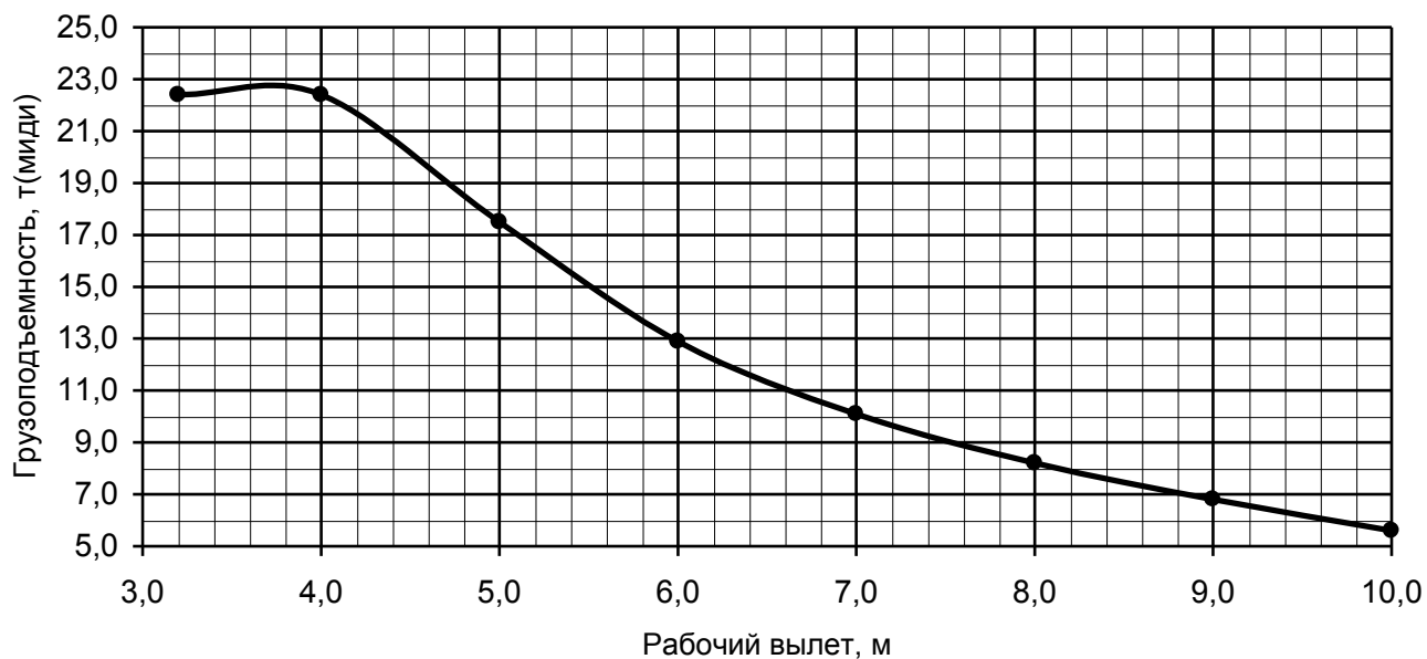
Грузовая характеристика L_{ст}=11,0-12,0 м. \kappa=10 противовес G=1,7 т.
