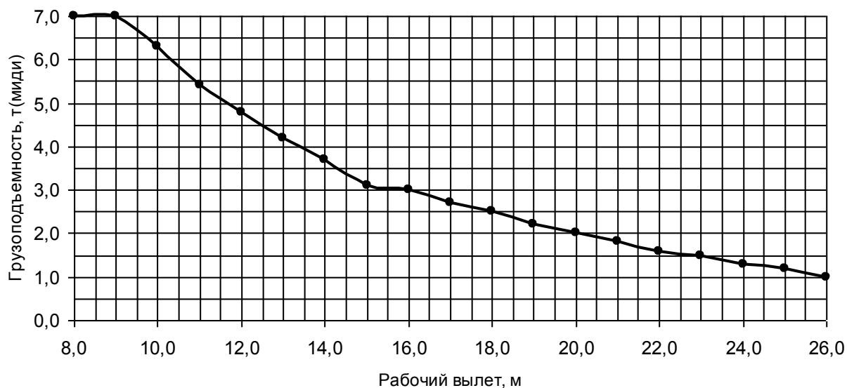
Грузовая характеристика. Лст=26,0-28,0м. к=4, противовес G=4,2 т.
