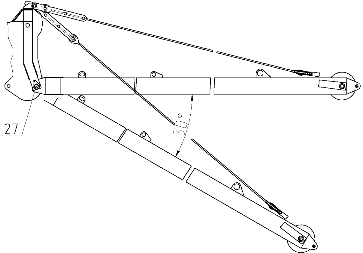
Рисунок 23 Удлинитель в рабочих положениях
