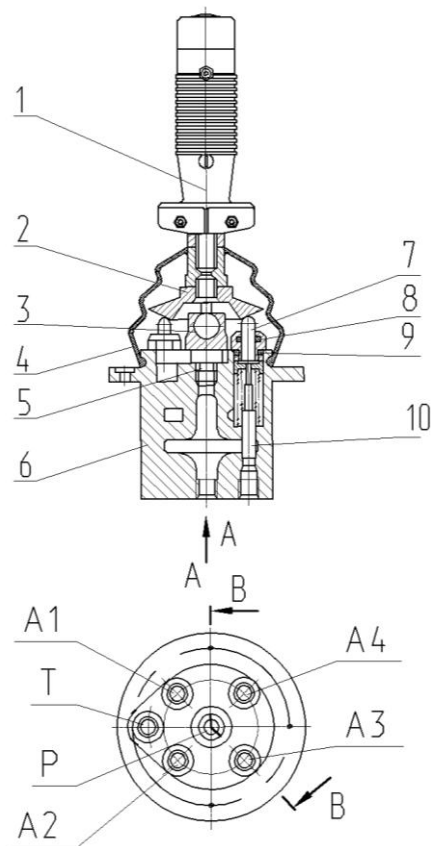
1 – рычаг; 2 – тарелка; 3 – шаровой шарнир; 4 – чехол; 5,9 – уплотнительные кольца; 6,12 – корпус блока; 7 – толкатель; 8 – манжета; 10 – золотник. P – подвод рабочей жидкости; T – сливное отверстие; A1 – A4 – рабочие отводы.
