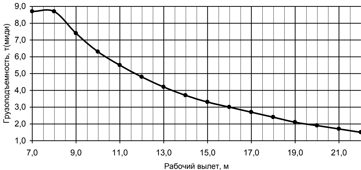
Грузовая характеристика. Лст=22,0-24,0м. κ=4, противовес G=4,2 т.
