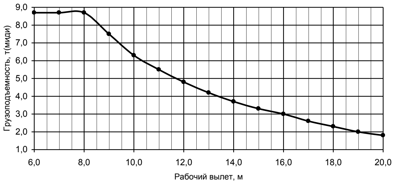
Грузовая характеристика. Лст=20,0-22,0м. κ=4, противовес G=4,2 т.
