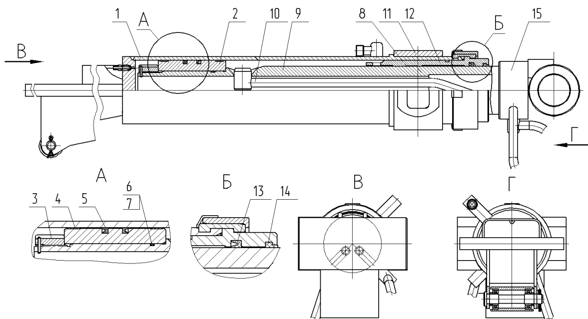
1 – гильза; 2 – поршень; 3 – гайка; 4 – кольцо направляющее; 5 – манжета; 6 – кольцо уплотняющее; 7 – втулка; 8 – кольцо направляющее; 9 – шток; 10 – трубопровод; 11 – цапфа гильзы; 12 – букса; 13 – кольцо уплотняющее; 14 – грязесъемник; 15 – цапфа штока; 16 – пробка
