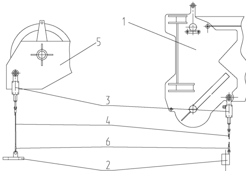
1- оголовок стрелы; 2- груз; 3- выключатель; 4- канат; 5- оголовок удлинителя; 6-зажим.
