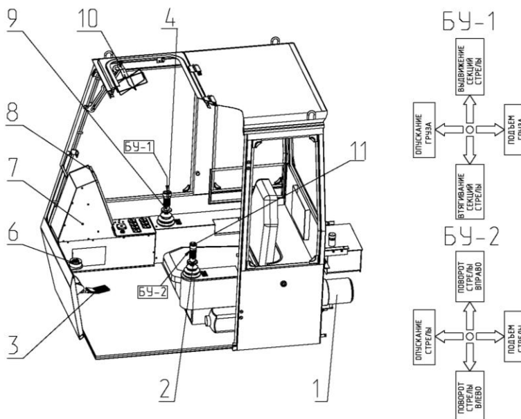
1 – отопительная установка; 2- рычаг блока управления рабочими операциями подъема-опускания стрелы и поворота поворотной рамы вправо и влево; 3 - педаль управления топливоподачей; 4 - кнопка управления ускорением лебедки; 6- креномер; 7 - пульт управления; 8- блок отображения информации (БОИ ОНК); 9 - рычаг управления грузовой лебедкой и выдвиганием втягивание секций стрелы; 10 – вентилятор; 11 – кнопка «звуковой сигнал».
