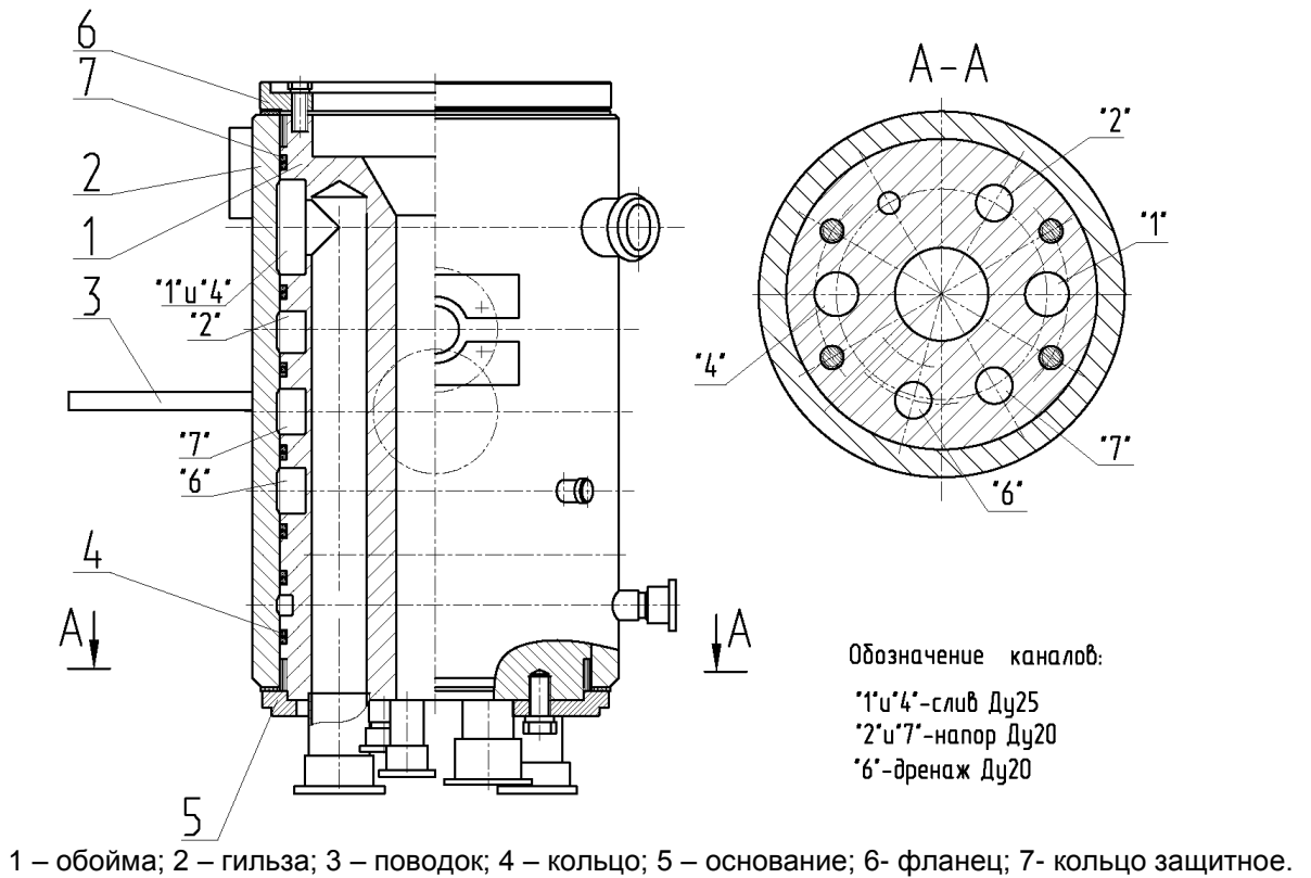
Рисунок 50 Центральный коллектор
