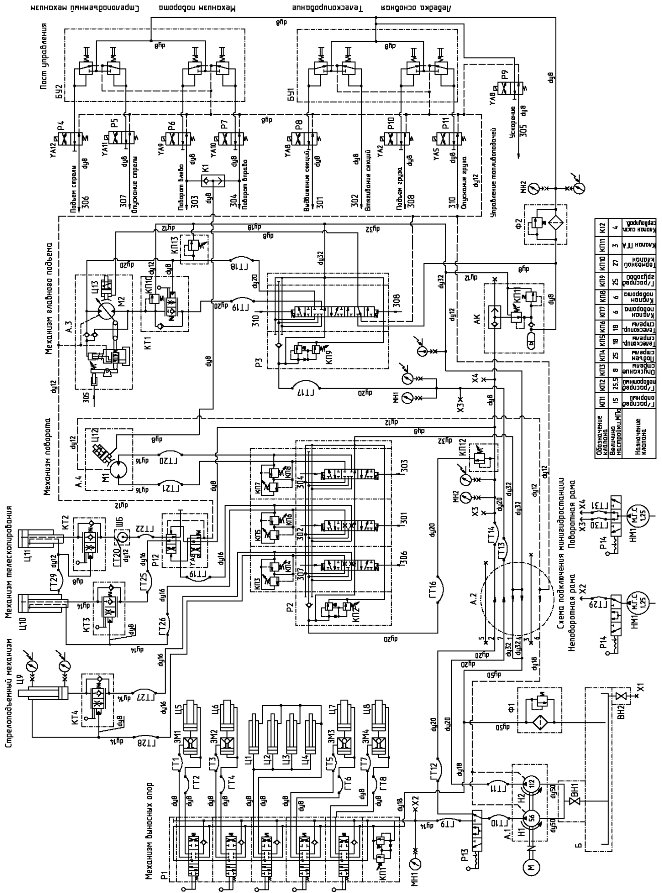
Рисунок 36 Схема гидравлическая принципиальная
