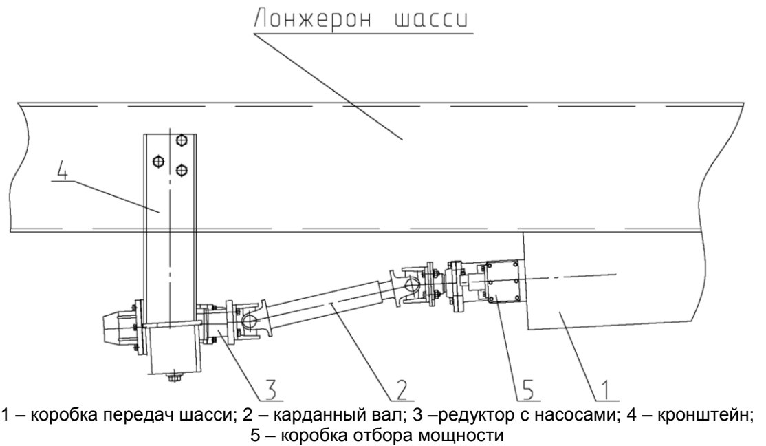
Рисунок 10 Установка привода насосов для шасси МАЗ 6303А3
