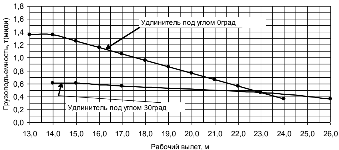
Грузовая характеристика. Лст=30,7м. к=1. Установлен удлинитель. Противовес G=1,7 т.
