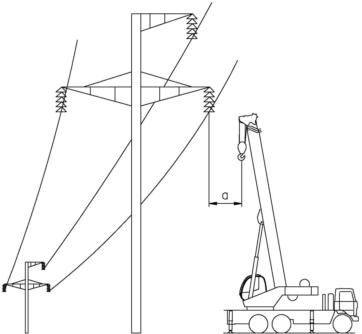
Рисунок 56 Схема установки крана вблизи линий электропередач
