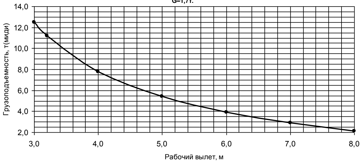
Грузовая характеристика Lст=9,9м. κ=10...12.Опорный контур 4,1x2,3м.,противовес G=1,7т.
