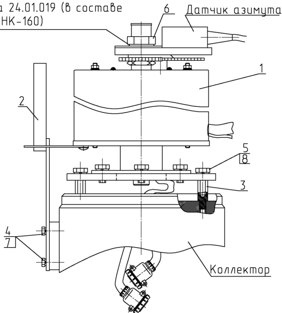
Рисунок 33 Токосъёмник
