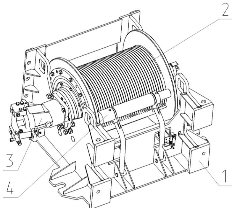
Рисунок 15 Рама поворотная с механизмами
