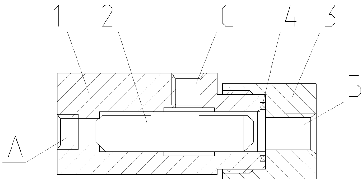
1- корпус; 2- золотник; 3- гайка; 4- уплотнение; А,В- напорные линии; С- к тормозу
