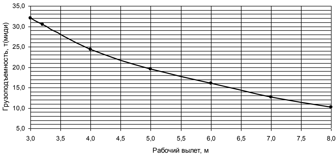
Грузовая характеристика. Лст=9,9м. к=12, противовес G=4,2 т.
