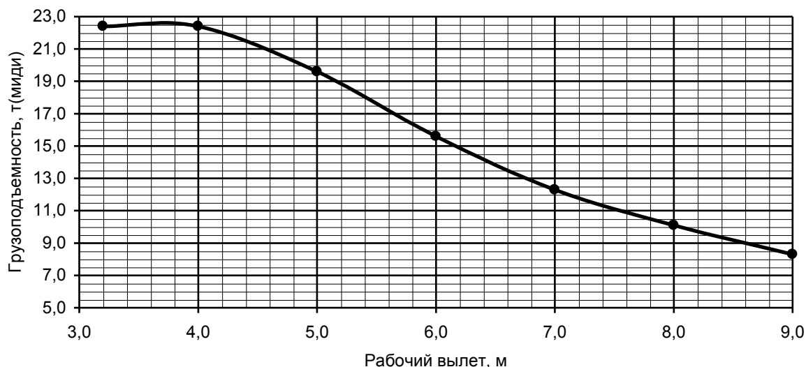
Грузовая характеристика. Лст=9,9-11,0м. κ=10 противовес G=4,2 т.
