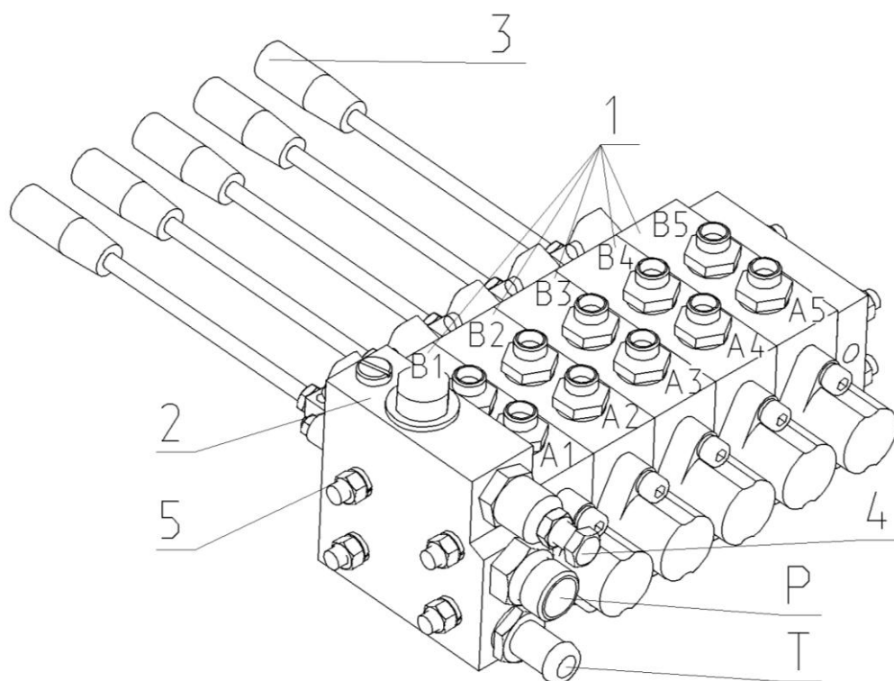
1- рабочая секция; 2- напорная секция; 3- рычаг; 4- клапан предохранительный; 5- шпилька A1-A5, B1-B5- рабочие отводы; P – напорный отвод; T – слив
