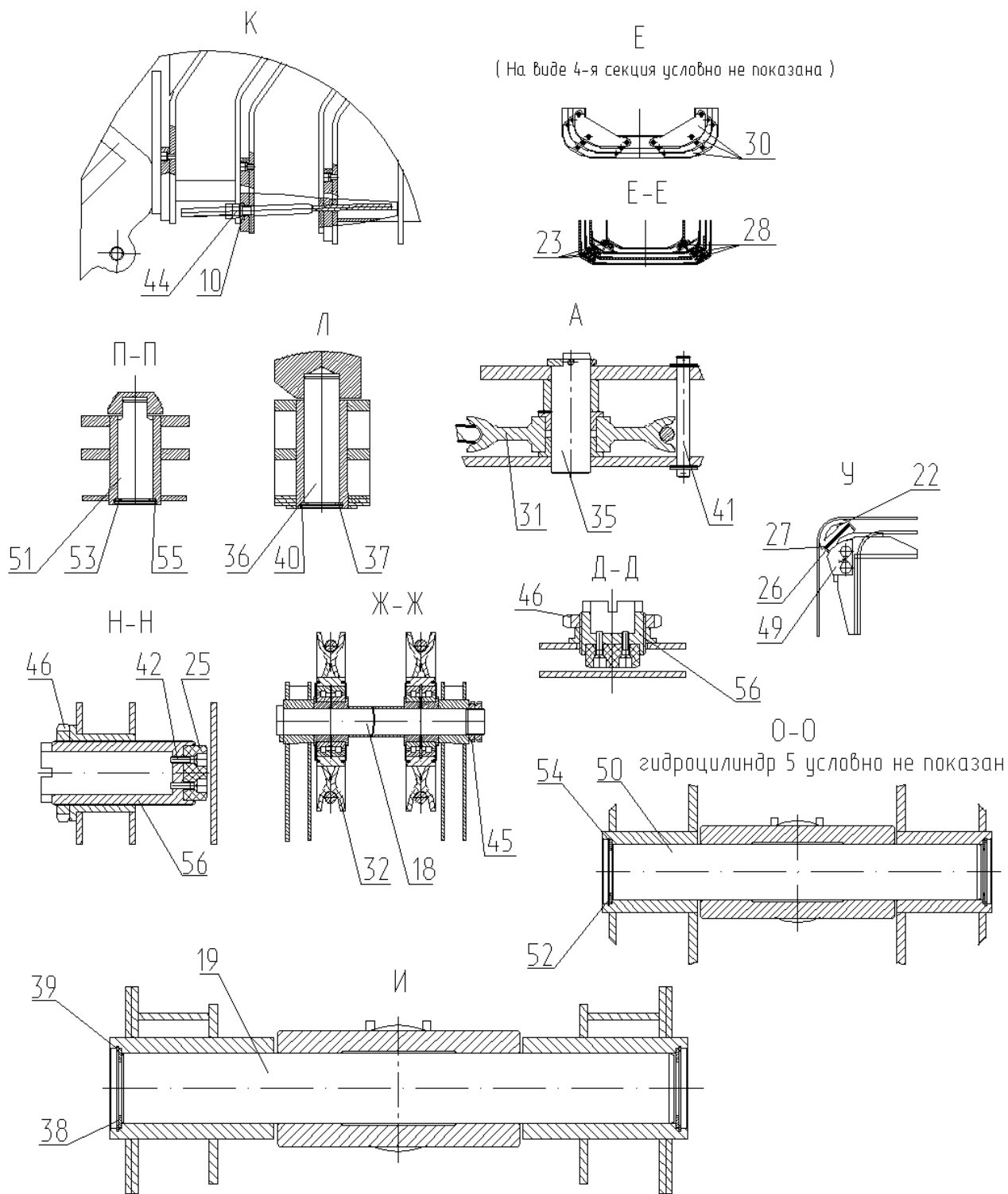
Рисунок 21.1 Стрела телескопическая
