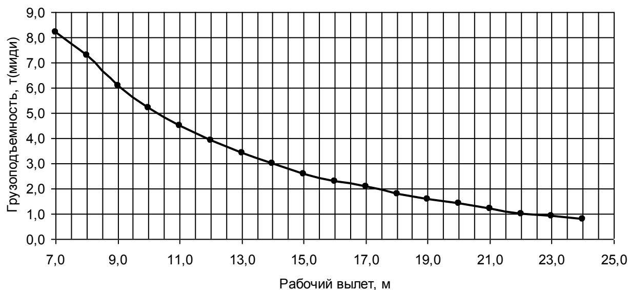
Грузовая характеристика L_{ст}=24,0-26,0 м. \kappa=4 , противовес G=1,7 т.
