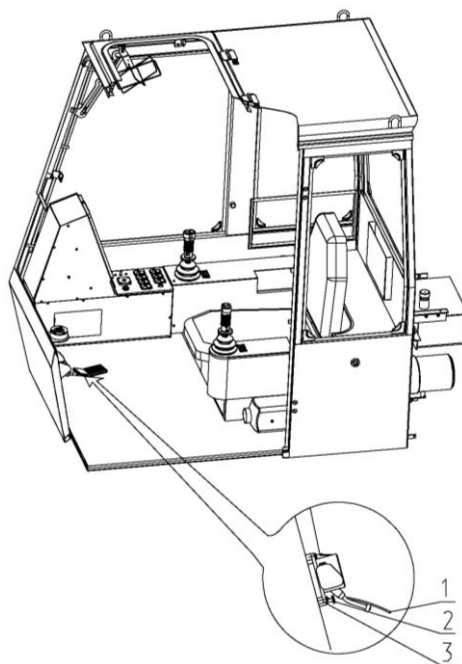
1- педаль управления топливоподачей; 2- винт; 3- контргайка.
