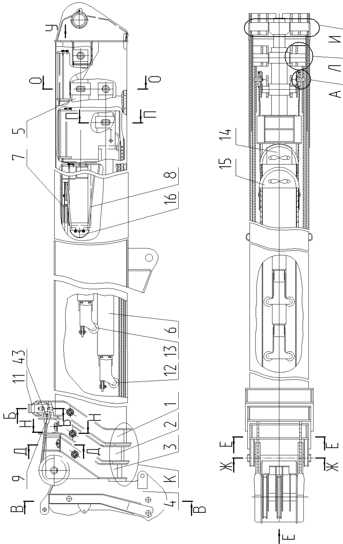
Рисунок 21 Стрела телескопическая (продолжение рис. 21.1, 21.2, 21.3, 21.4)
