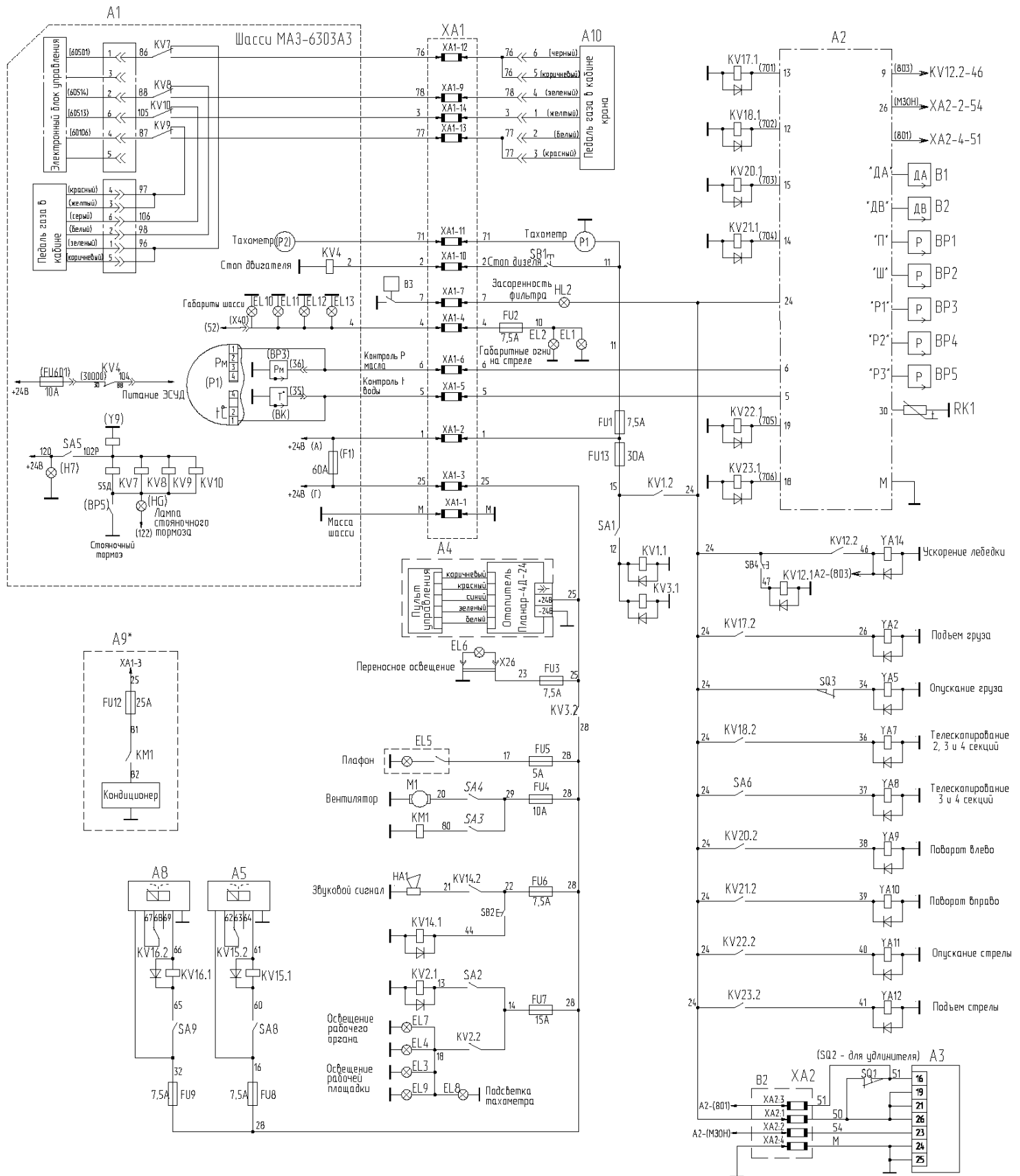
Рисунок 29 Схема электрическая принципиальная (шасси MA3-6303A3)
