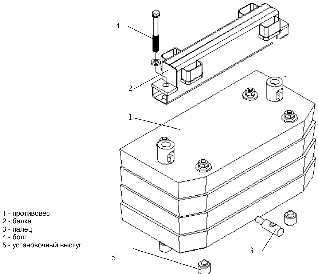
Рисунок 27 Установка дополнительного противовеса
