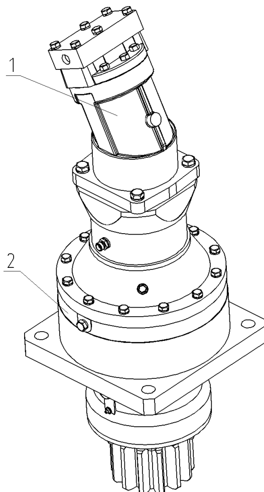
1-гидромотор, 2-редуктор
