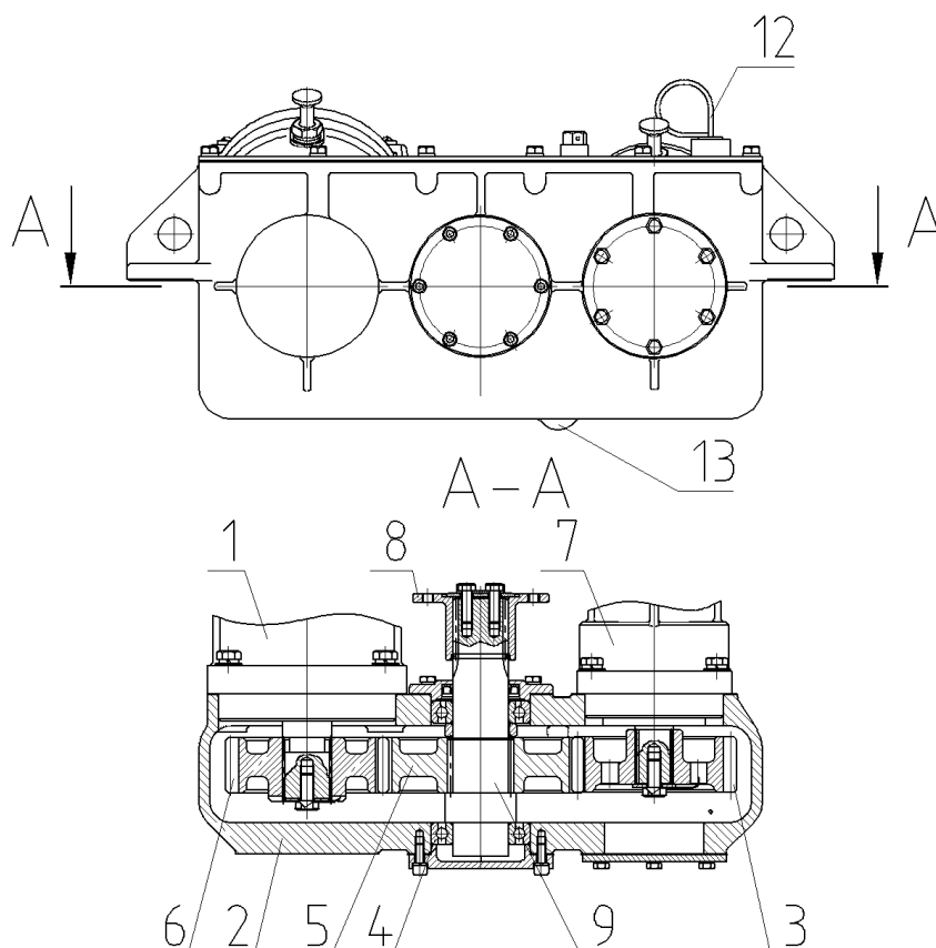
1,7 – аксиально - поршневые насосы; 2 – корпус; 3 – зубчатое колесо; 4 - подшипник; 5 - зубчатое колесо; 6 - зубчатое колесо; 8 – фланец; 9 – вал; 12 – масломер; 13 – пробка
