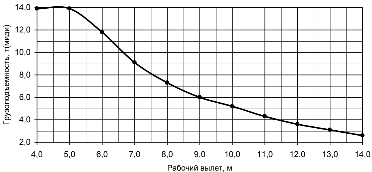
Грузовая характеристика L_{ст}=14,0-16,7м. κ=10 , противовес G=1,7 т.
