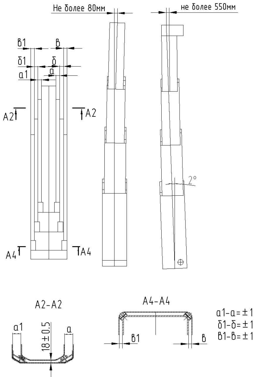
Рисунок 21.4 Схема регулировок отклонения секции от продольной оси
