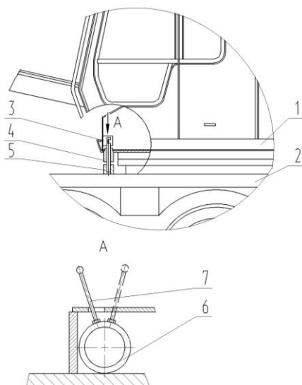
1 – поворотная рама; 2 – неповоротная рама; 3 – пластина; 4,5 – втулка; 6 – штырь; 7 - ручка
