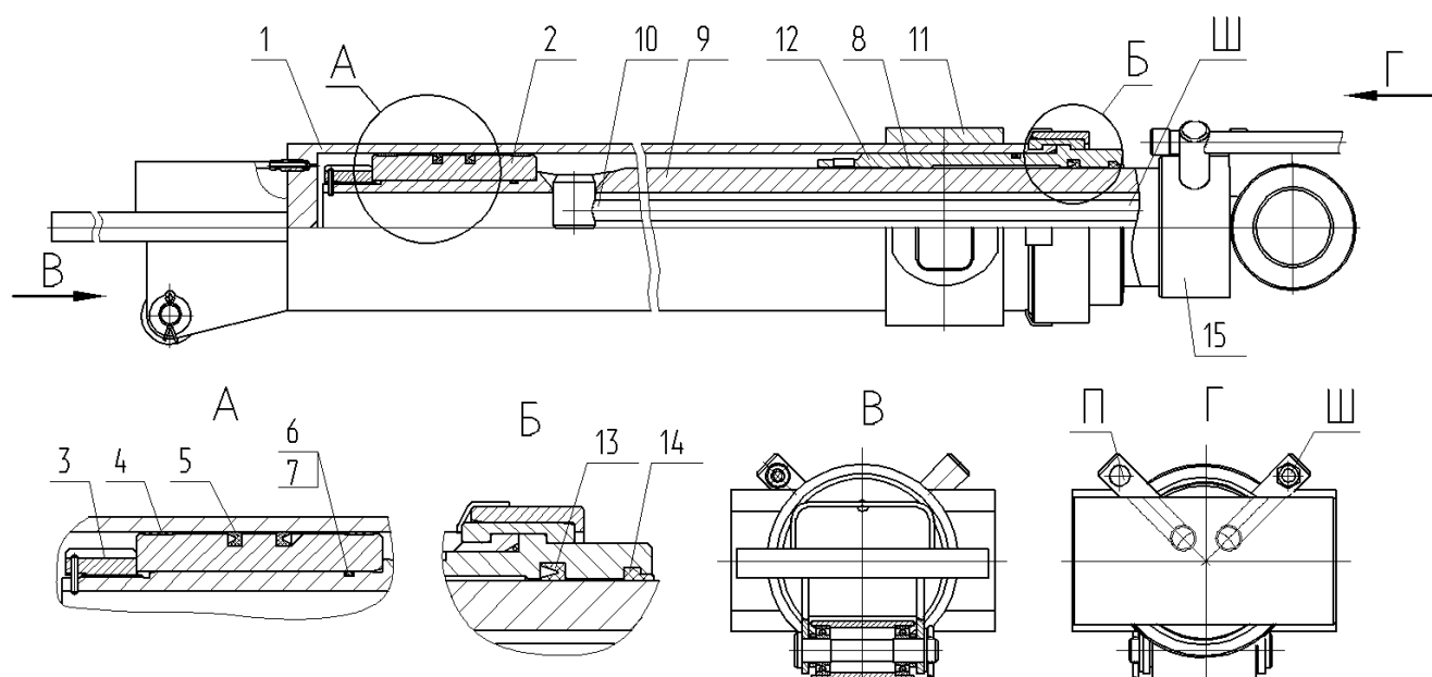
1 – гильза; 2 – поршень; 3 – гайка; 4 – кольцо направляющее; 5 – манжета; 6 – кольцо уплотняющее; 7 – втулка; 8 – кольцо направляющее; 9 – шток; 10 – трубопровод; 11 – цапфа гильзы; 12 – букса; 13 – кольцо уплотняющее; 14 – грязесъемник; 15 – цапфа штока; 16 – пробка Ш – отверстие штоковой полости; П – отверстие поршневой полости.
