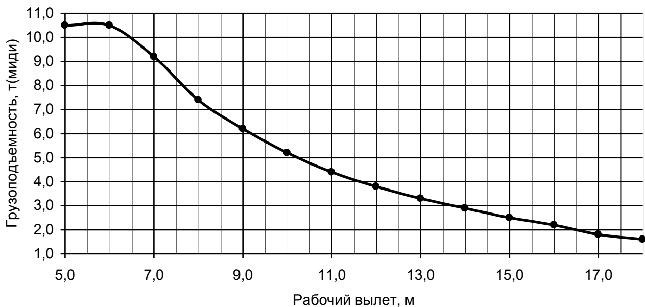
Грузовая характеристика L_{ст}=18,0-20,0м. κ=4 , противовес G=1,7 т.
