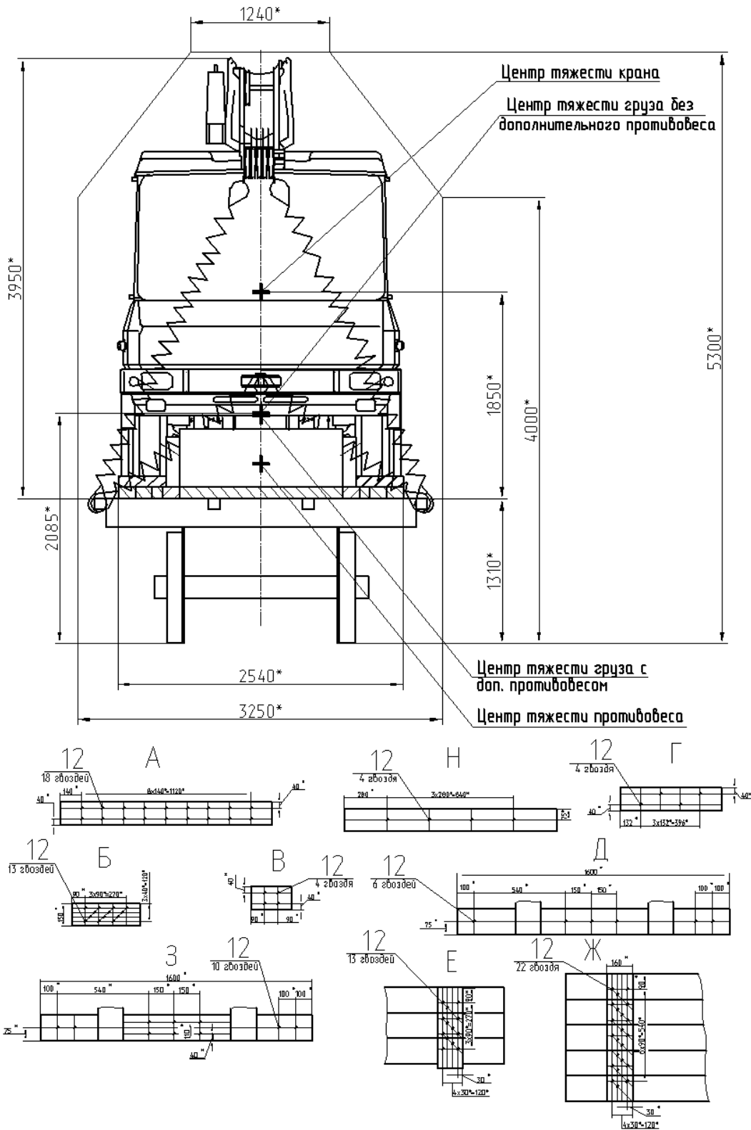
Рисунок 66 Схема отгрузки крана
