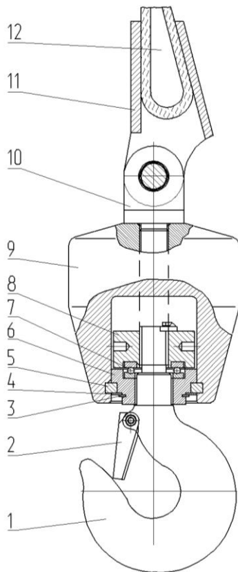
1 – крюк; 2 – защелка; 3 – кольцо; 4 – шайба; 5 – сухарь; 6 – опора; 7 – подшипник; 8 – гайка; 9 – груз; 10 – тяга; 11 – втулка клиновья; 12 – клин
