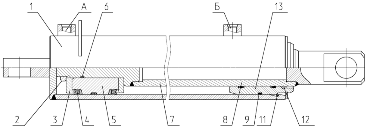
11 – корпус; 2 – гайка; 3 – шайба; 4 – манжета; 5 – поршень; 6 – кольцо; 7 – шток; 8,9 – кольца; 11 – кольцо стопорное; 12 – грязесъемник; 13 – гильза А- отверстие поршневой полости; Б- отверстие штоковой полости.
