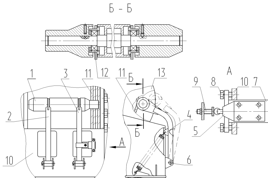
1-ролик; 2, 3-кронштейны; 4-пружина; 5-конечный выключатель; 6-ось; 7-кронштейн; 8-болт; 9-винт; 10-рама; 11-канат; 12-подшипник; 13-барабан
