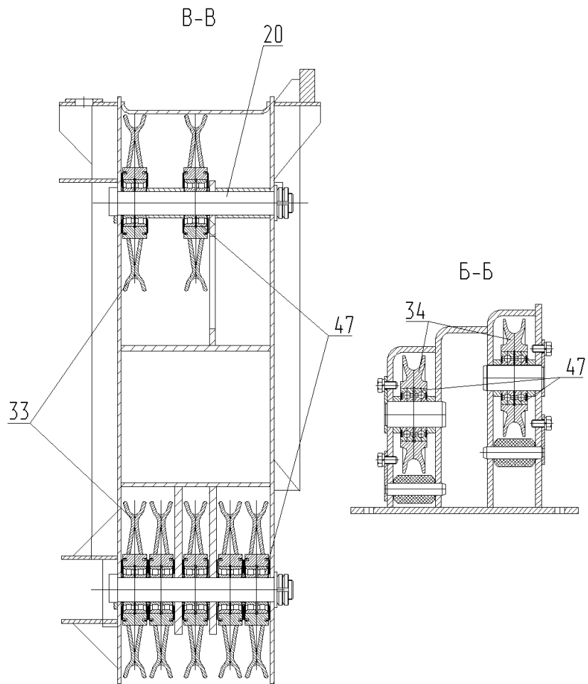
Рисунок 21.2 Стрела телескопическая
