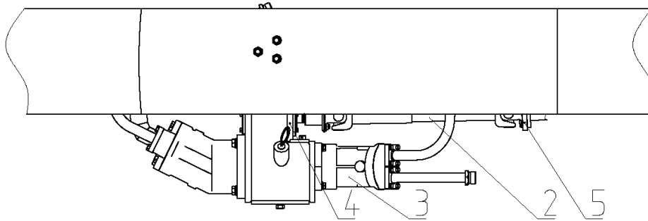
Рисунок 10 Установка привода насосов для шасси МАЗ 6303А3
