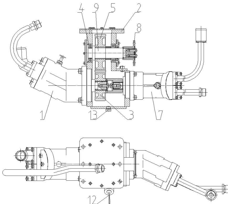
1,7 – аксиально - поршневые насосы; 2 – корпус; 3 – зубчатое колесо; 4 - подшипник; 5 - зубчатое колесо; 6 - зубчатое колесо; 8 – фланец; 9 – вал; 12 – масломер; 13 – пробка
