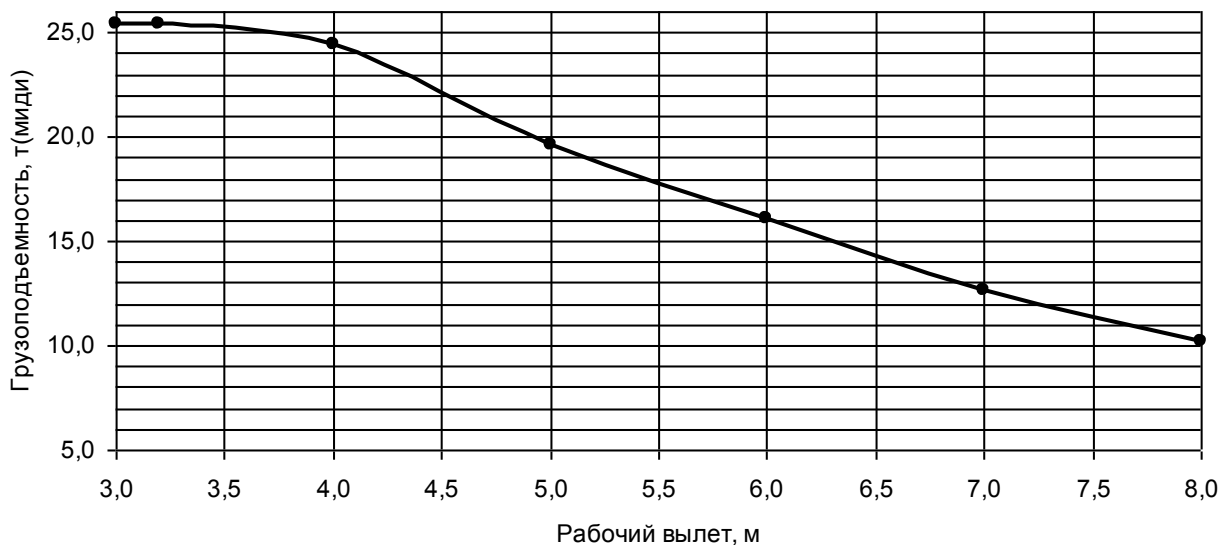
Грузовая характеристика. Лст=9,9м. к=10, противовес G=4,2 т.
