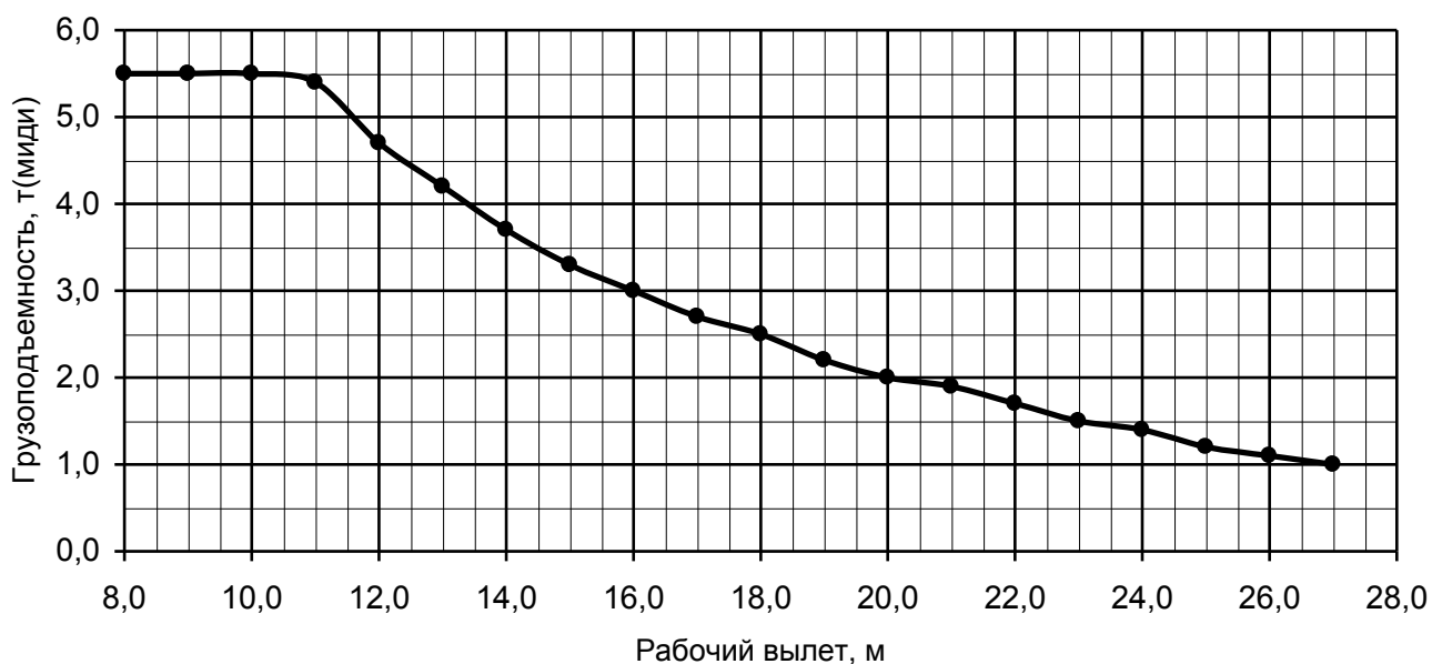
Грузовая характеристика Лст=9,9м. к=10...12. Опорный контур 4,1x2,3м., противовес G=4,2т.
