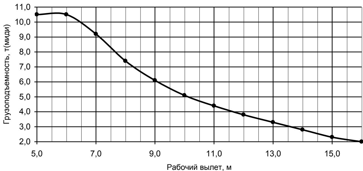
Грузовая характеристика L_{ст}=16,7-18,0м. κ=4 , противовес G=1,7 т.
