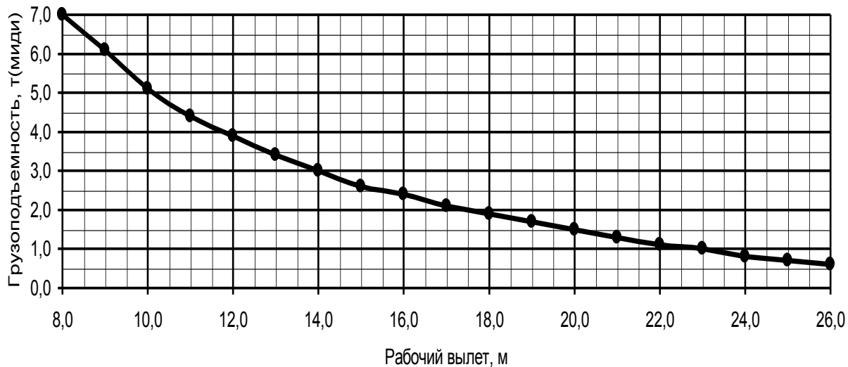
Грузовая характеристика. Lст=26,0-28,0м. κ=4, противовес G=1,7 т.
