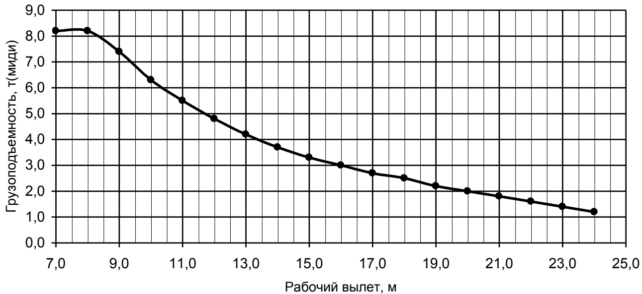
Грузовая характеристика. Лст=24,0-26,0м. κ=4, противовес G=4,2 т.
