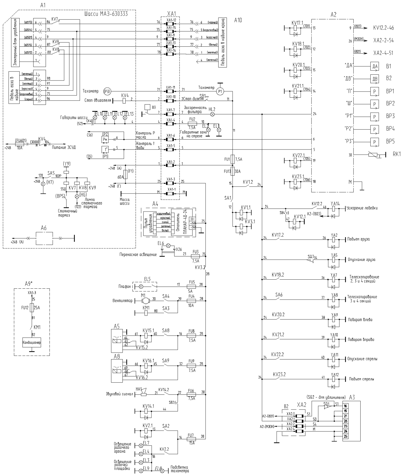
Рисунок 30 Схема электрическая принципиальная (шасси МА3-630333)
