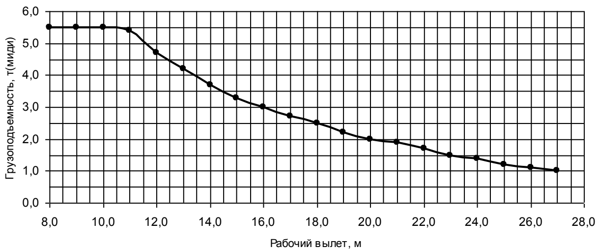
Грузовая характеристика Lст=9,9м. κ=10...12.Опорный контур 4,1x2,3м.,противовес G=1,7т.
